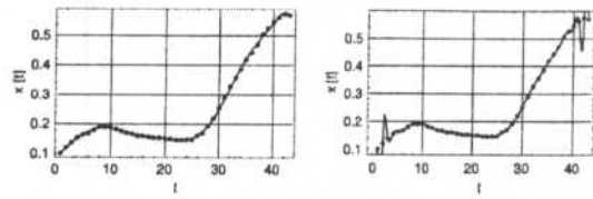
Abbildung 10: links: x(t) mit n = 10 , rechts: n = 30
